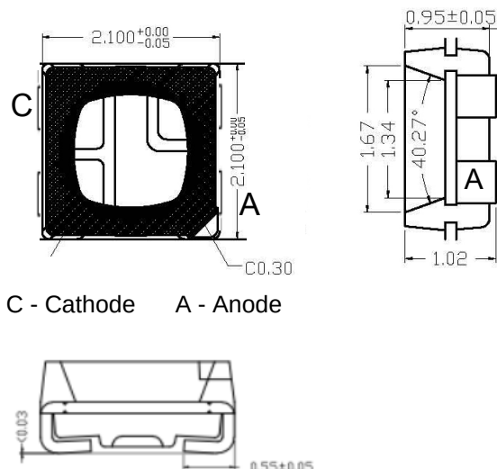
Top Side
