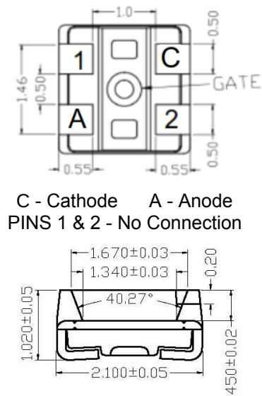
Bottom Side
