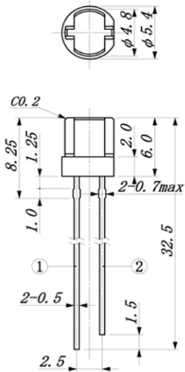
① Anode
